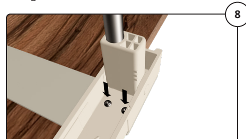
8 Innere Schrauben (M3x8) festdrehen (auf beiden Seiten).
