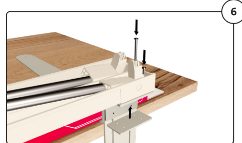
6 Die äußeren Schrauben (M3x8 und M3x45) festdrehen und dabei die Gewindeplatte von unten andrücken (Auf beiden Seiten).
