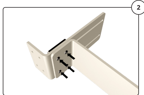
2 Schrauben (M3x10) hinein drehen, aber noch nicht festdrehen. (x2)
